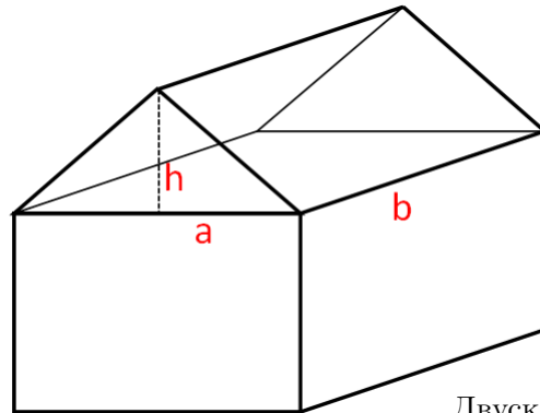
Двускатная крыша
